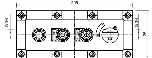
MUML
